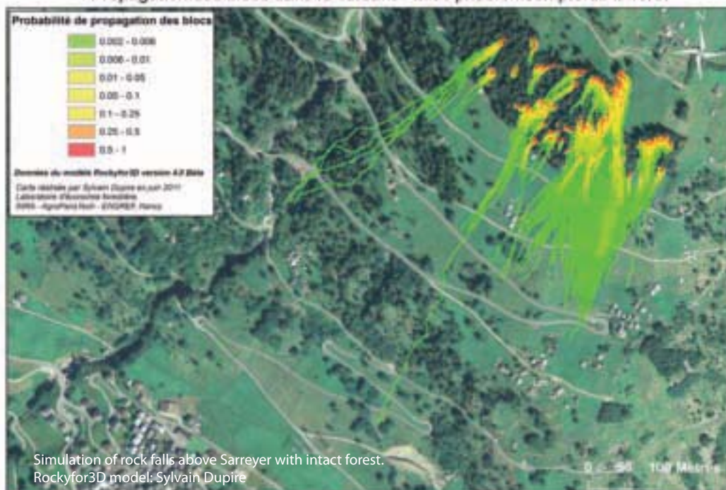
Propagation des blocs dans le versant - avec prise en compte de la forêt
